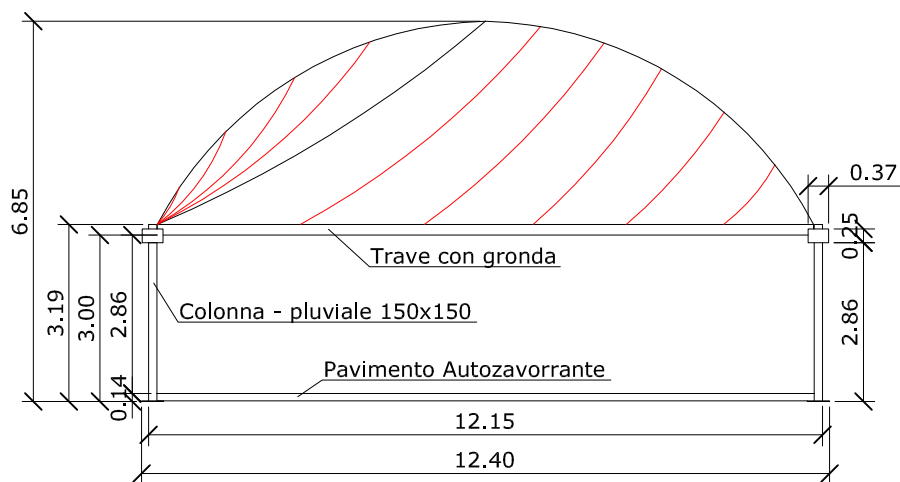
- PROSPETTO
