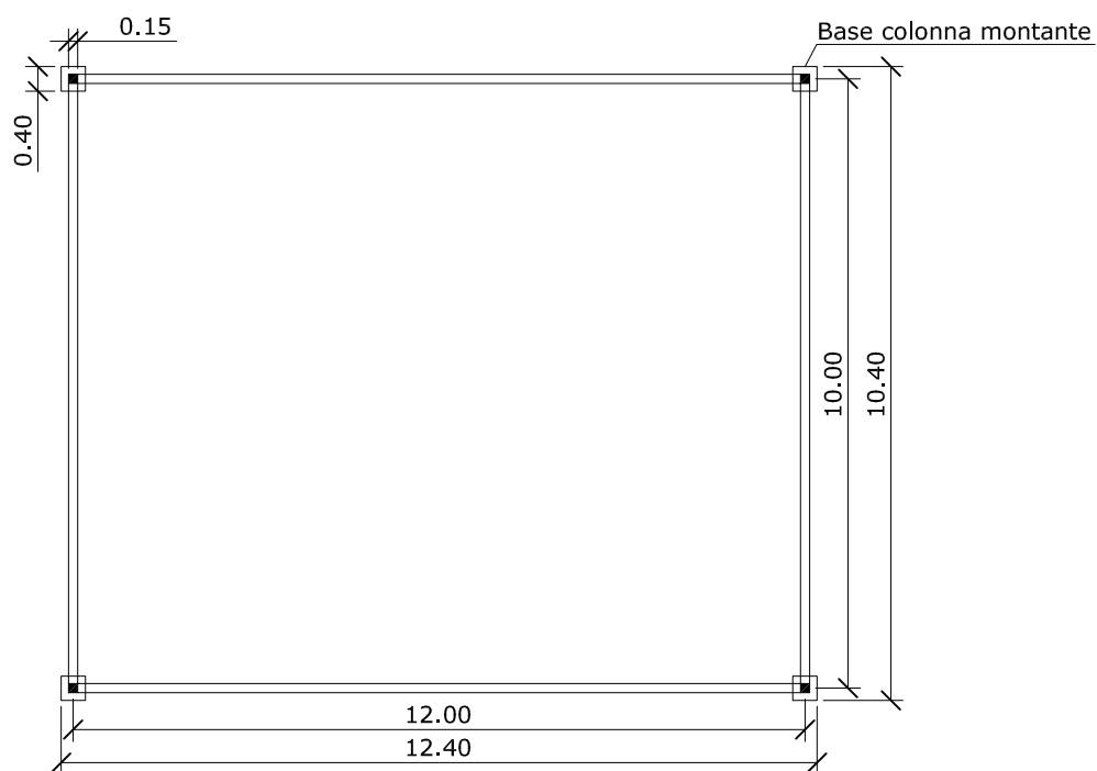
- PIANTA
